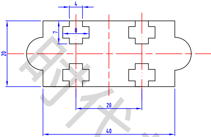
导柱截面图:
